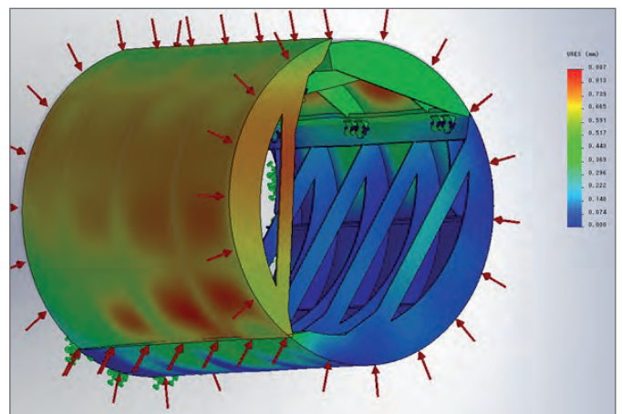
Verformungs- und Steifigkeitsberechnung mittels 3D-Finite-Elemente Nachweisverfahren
