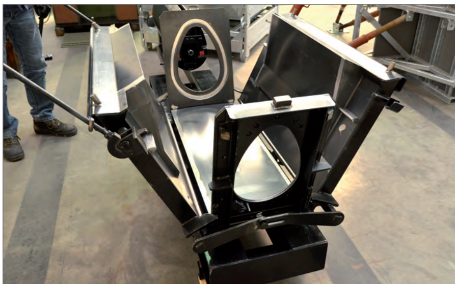
Bei Auf- und Zuklappen der Seitenelemente bewegen sich alle Elemente zwangsgeführt gleichzeitig. Die Rinne ist nun ausgeschalt und kann entnommen werden.
